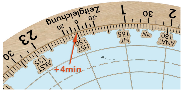
Bild 14: Einstellung der Zeitgleichung für den 15. Mai (+4 min)
