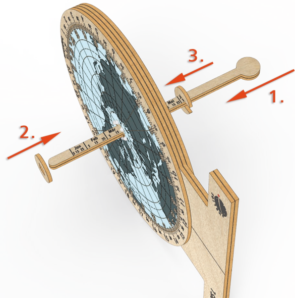
Bild 11: Der Schattenwerfer wird von unten durch die rechteckige Aussparung gesteckt und mit den Abdeckungen oben und unten befestigt.
