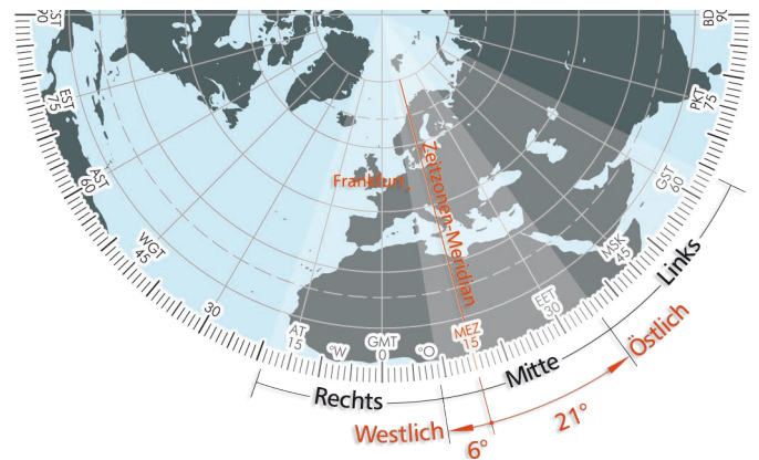
Bild 6: Die Position des Zeiringträgers in Bild 5 richtet sich nach der Lage des Standorts relativ zum Zeitzonen-Meridian.
