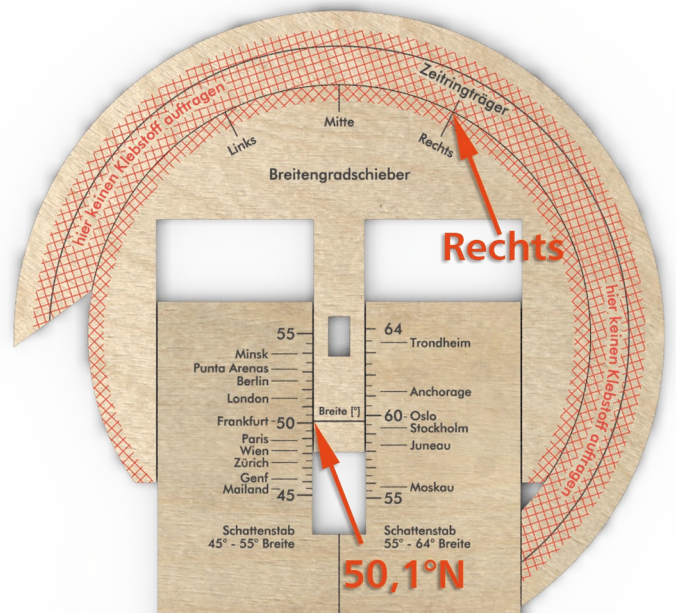
Bild 5: Der Breitengradschieber wird auf die Breite des Standorts (hier Frankfurt 50,1°N) eingestellt. Der Zeiringträger schlägt rechts an.
