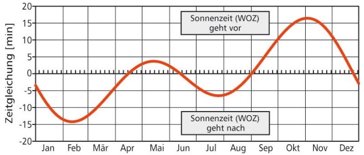
Bild 2: Zeitgleichung
