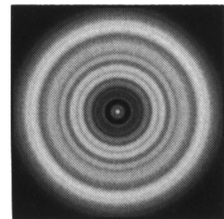
Figura 6-1 Un telescopio colimado aparecerá como una formación simétrica en forma de aro similar al disco de difracción que se ve aquí.
